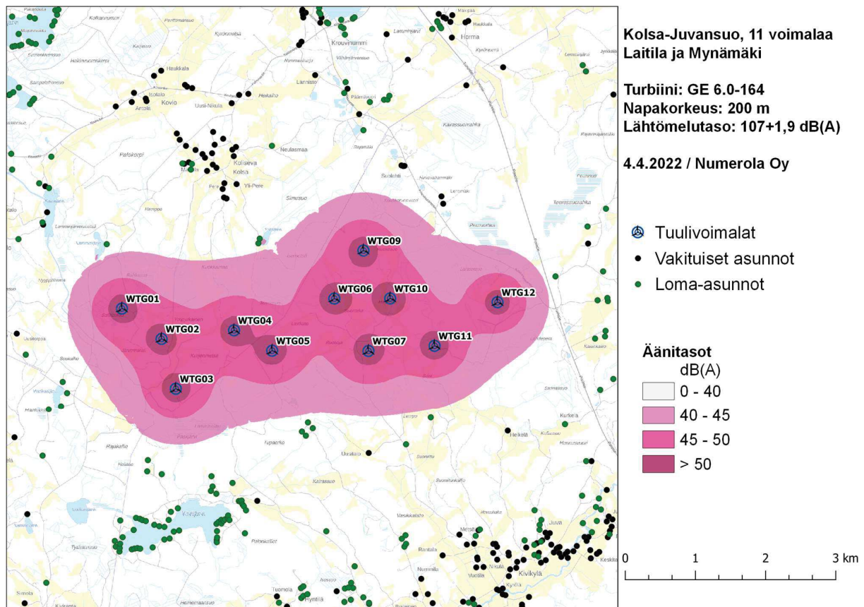
Kuva 18. Kartta melun leviämisestä Kolsa-Juvansuon tuulivoimapaiston alueella (VE2).
