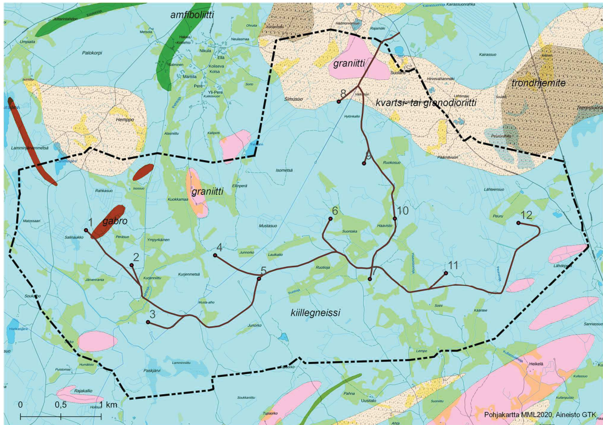
Kuva 98. Hankealueen kallioperä.
