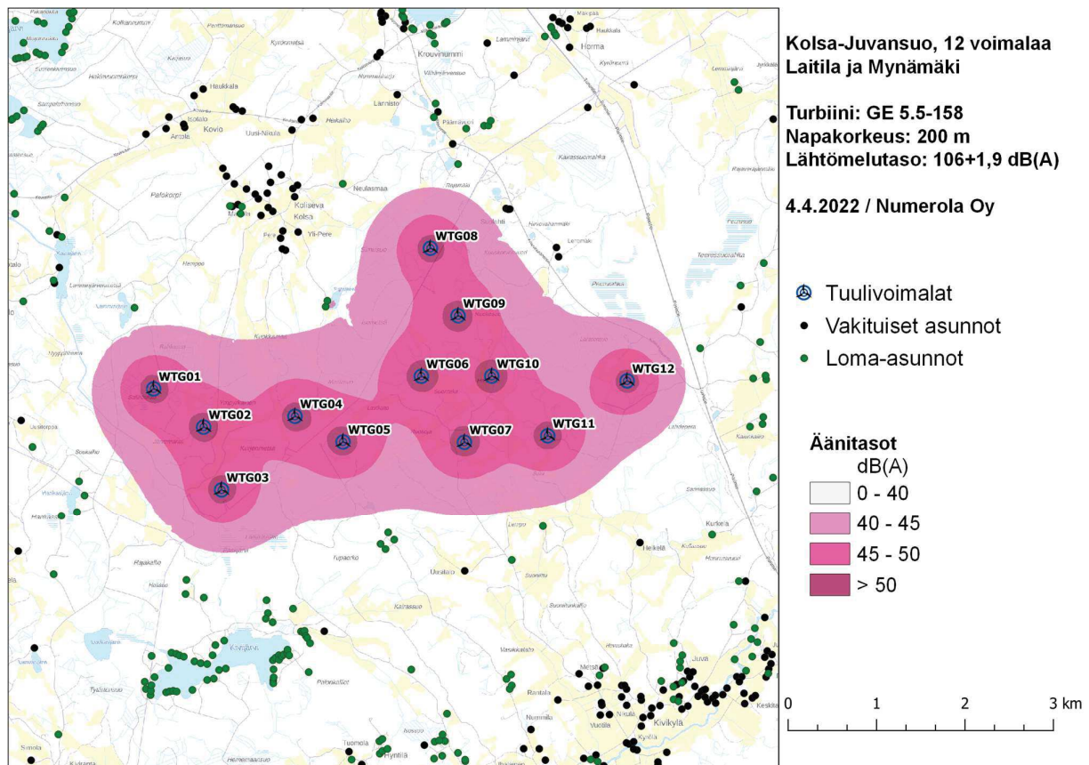
Kuva 17. Kartta melun leviämisestä Kolsa-Juvansuon tuulivoimapaiston alueella (VE1).
