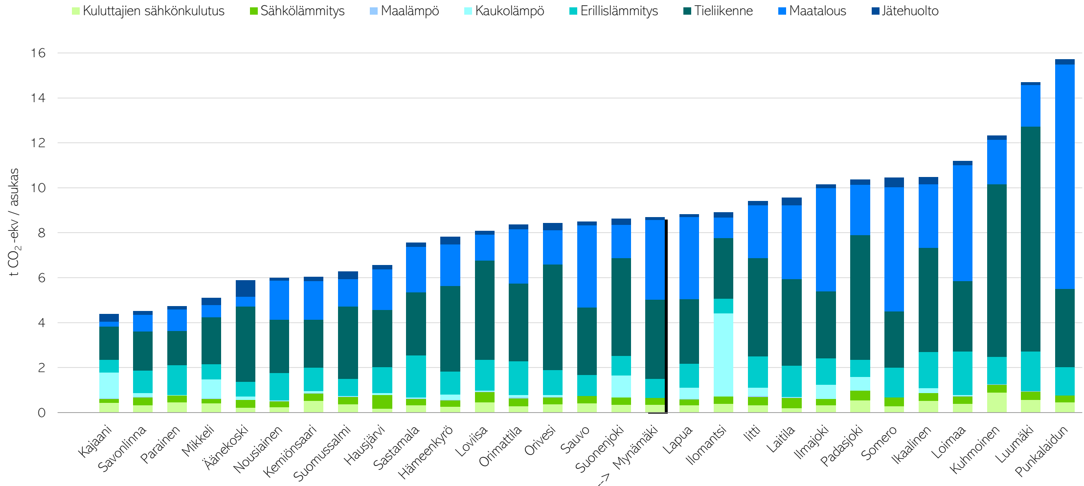
Kuva 11. Asukaskohtaisten päästöjen (t CO 2 -ekv/asukas) vertailu (ilman teollisuutta) vuonna 2021 sellaisissa CO 2 -raportin kunnissa, joissa on alle 25 asukasta maaneliökilometrillä.
