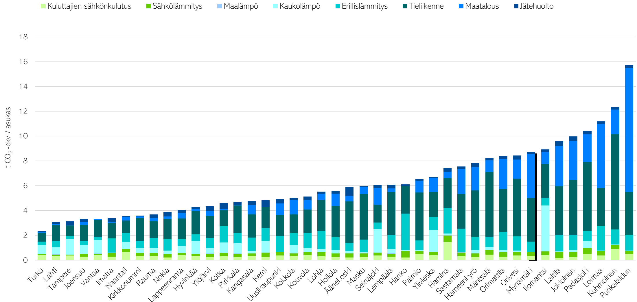
Kuva 13. CO2-raportissa mukana olevien Hinku-kuntien asukaskohtaiset päästöt (t CO 2 -ekv/asukas) sektoreittain vuonna 2021. Teollisuuden päästöt eivät ole mukana tarkastelussa.
