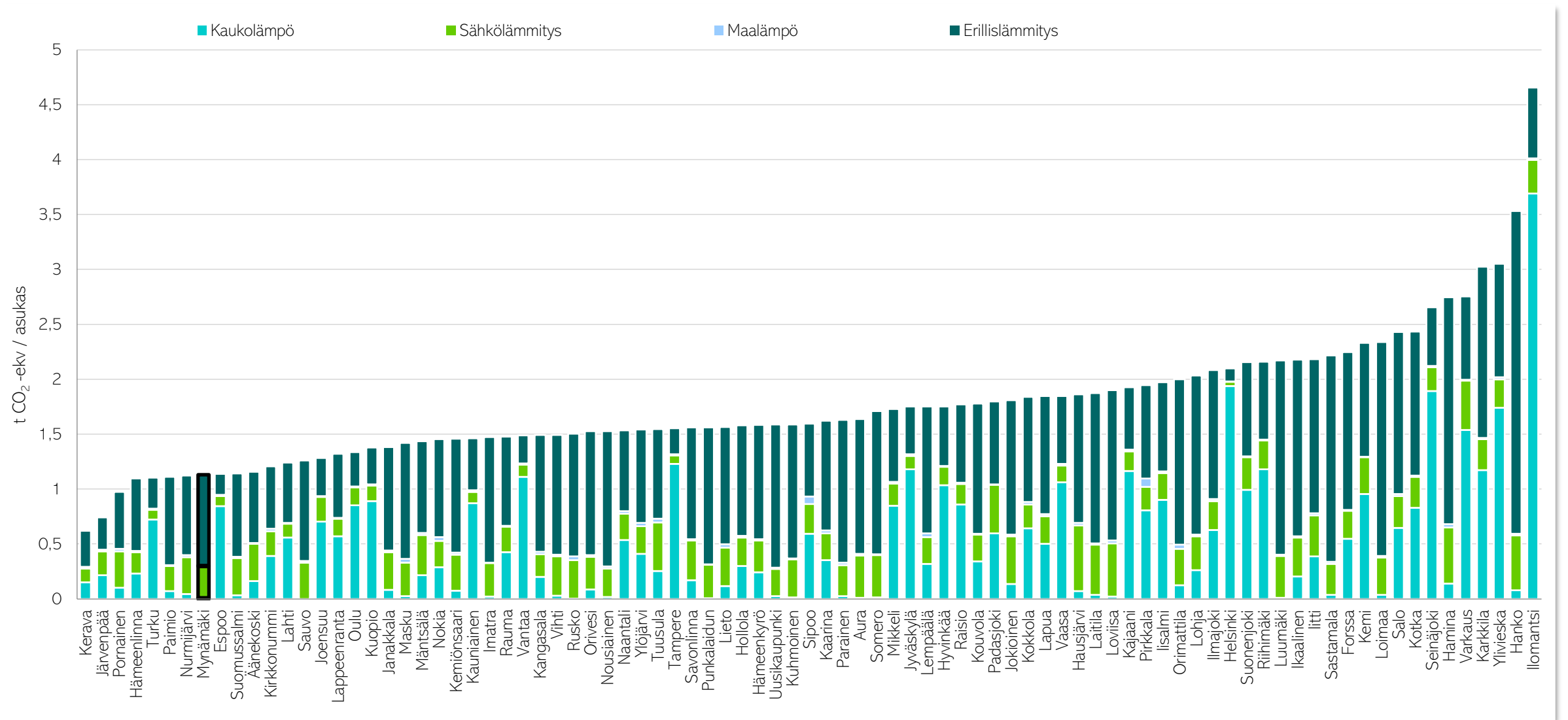
Kuva 16. Asukaskohtaiset päästöt (t CO 2 -ekv/asukas) lämmityksestä kaikissa CO 2 -raportin kunnissa vuonna 2021.
