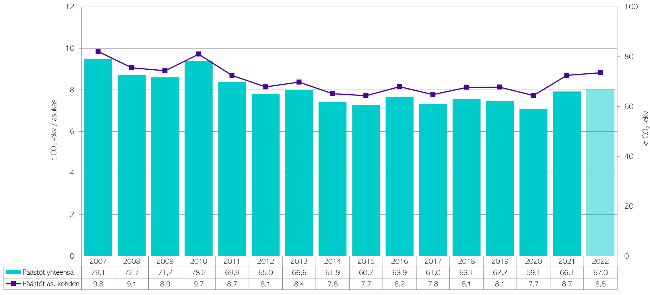
Kuva 3. Päästöt yhteensä ja asukasta kohden Mynämäellä vuosina 2007–2022 ilman teollisuutta. Vuoden 2022 tieto on ennakkotieto.
