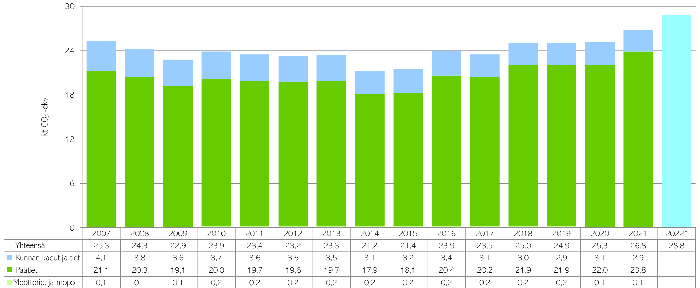
Kuva 6. Tieliikenteen päästöt Mynämäellä vuosina 2007–2022. Vuoden 2022 tieto on ennakkotieto, joka perustuu muutoksiin liikennepolttoaineiden jakeluvelvoitteessa.
