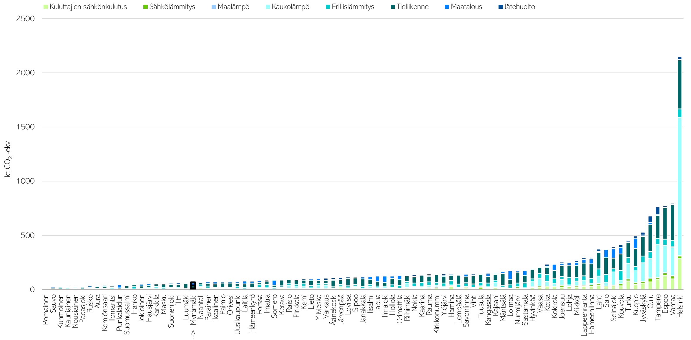
Kuva 17. Kokonaispäästöt (kt CO 2 -ekv) kaikissa CO 2 -raportin kunnissa vuonna 2021 ilman teollisuutta.
