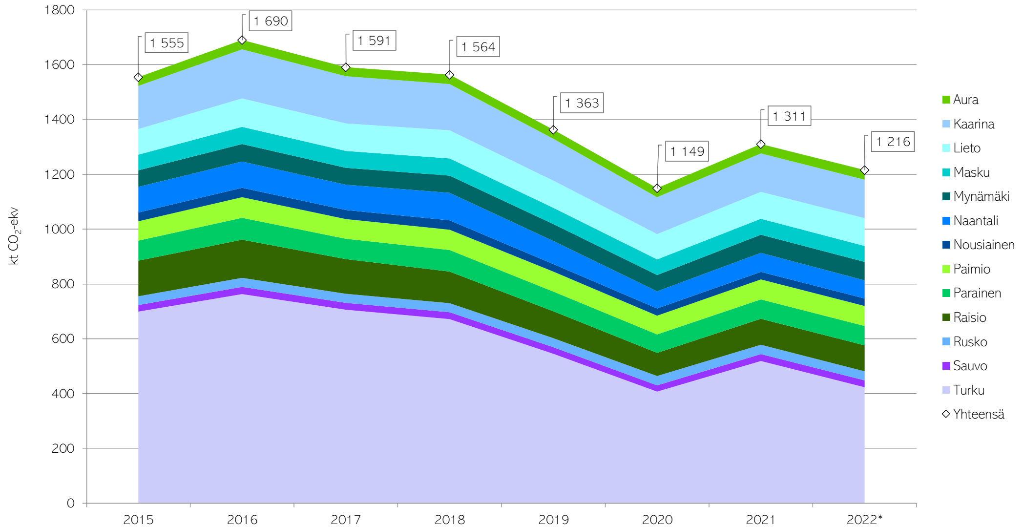
Kuva 12. Turun kaupunkiseudun kuntien kasvihuonekaasupäästöt yhteensä vuosina 2015–2022. Vuoden 2022 tieto on ennakkotieto. Teollisuuden päästöt eivät ole mukana tarkastelussa. Kasvihuonekaasupäästöt ovat TKS-kuntien yksi MAL-sopimuksen vaikuttavuuden indikaattori.
